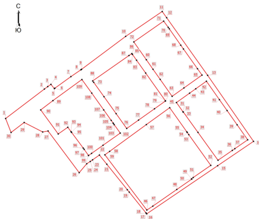
Схема границ полигона ДМ-05-1, вырез (внутренний контур):
